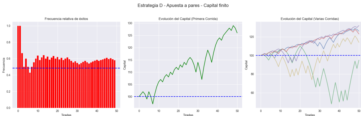
Figura 4: Gráficas de Frecuencia Relativa y Flujo de Capital bajo una Estrategia de Apuesta D'Alembert
